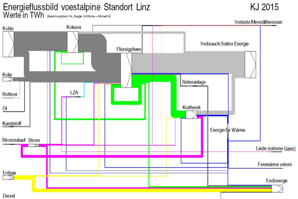
Abbildung 3 Energieflüsse im Stahlwerk der voestalpine mit der vorgelagerten Kokerei am Standort Linz
